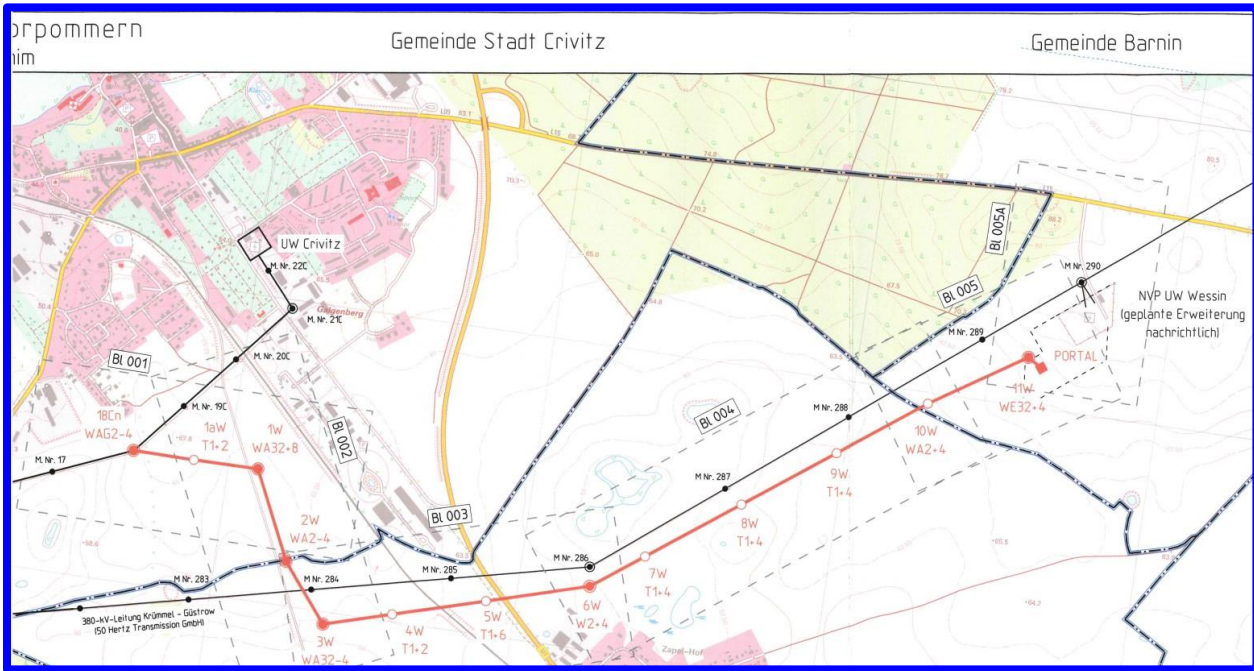
Karte – Verlauf 110-kV Hochspannungsfreileitung
